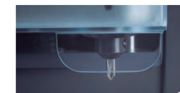
7 Schutzverkleidung für Späne Écran protecteur de copeaux
